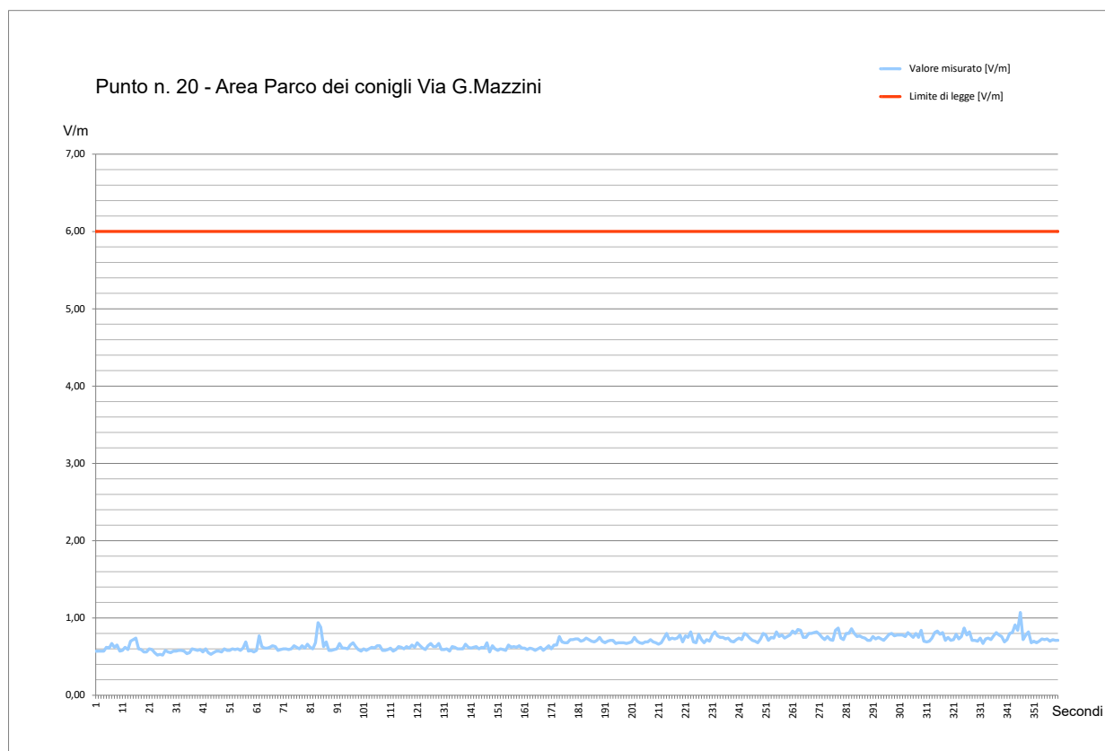
Fig. 67 Grafico Misura di Campo Elettromagnetico a RadioFrequenza – Punto #20
