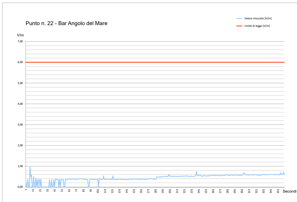
Fig. 73 Grafico Misura di Campo Elettromagnetico a RadioFrequenza – Punto #22
