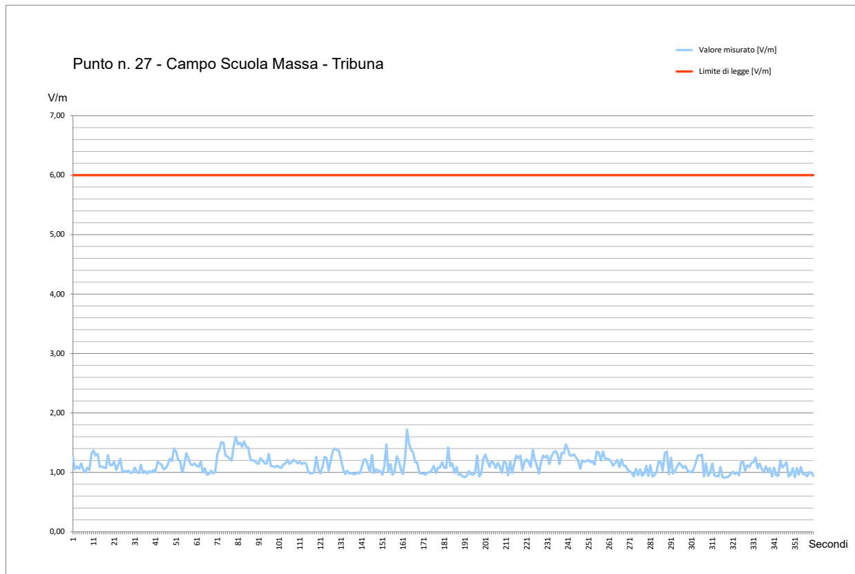
Fig. 88 Grafico Misura di Campo Elettromagnetico a RadioFrequenza – Punto #27
