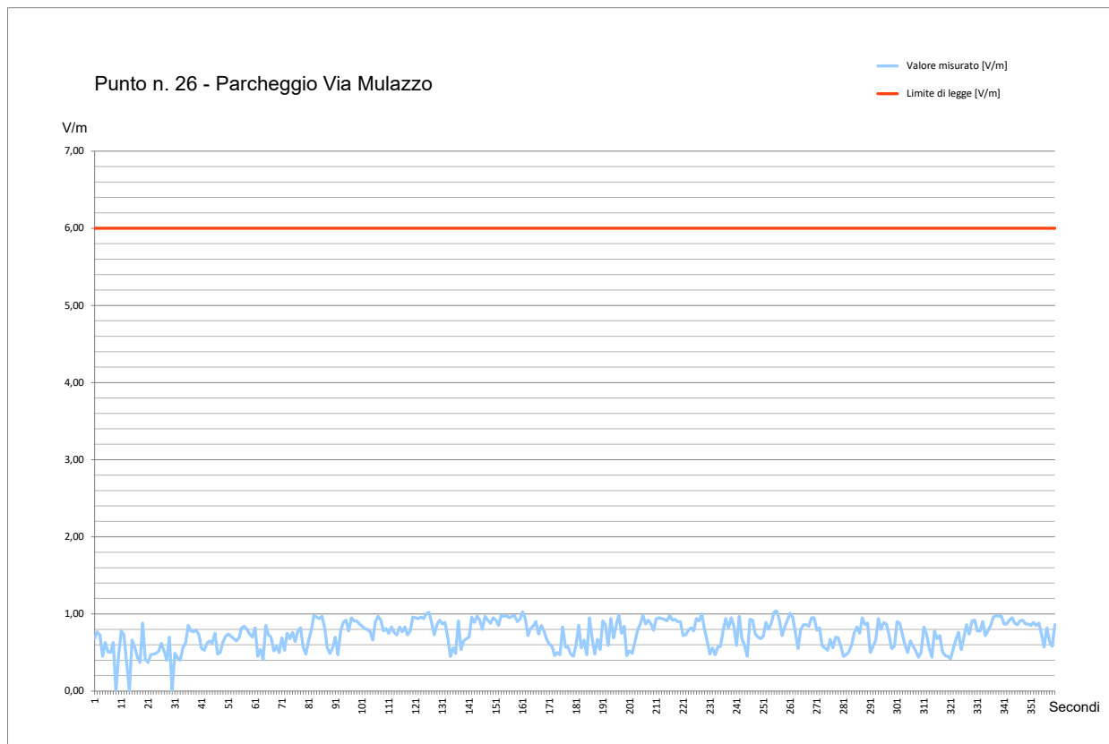
Fig. 85 Grafico Misura di Campo Elettromagnetico a RadioFrequenza – Punto #26
