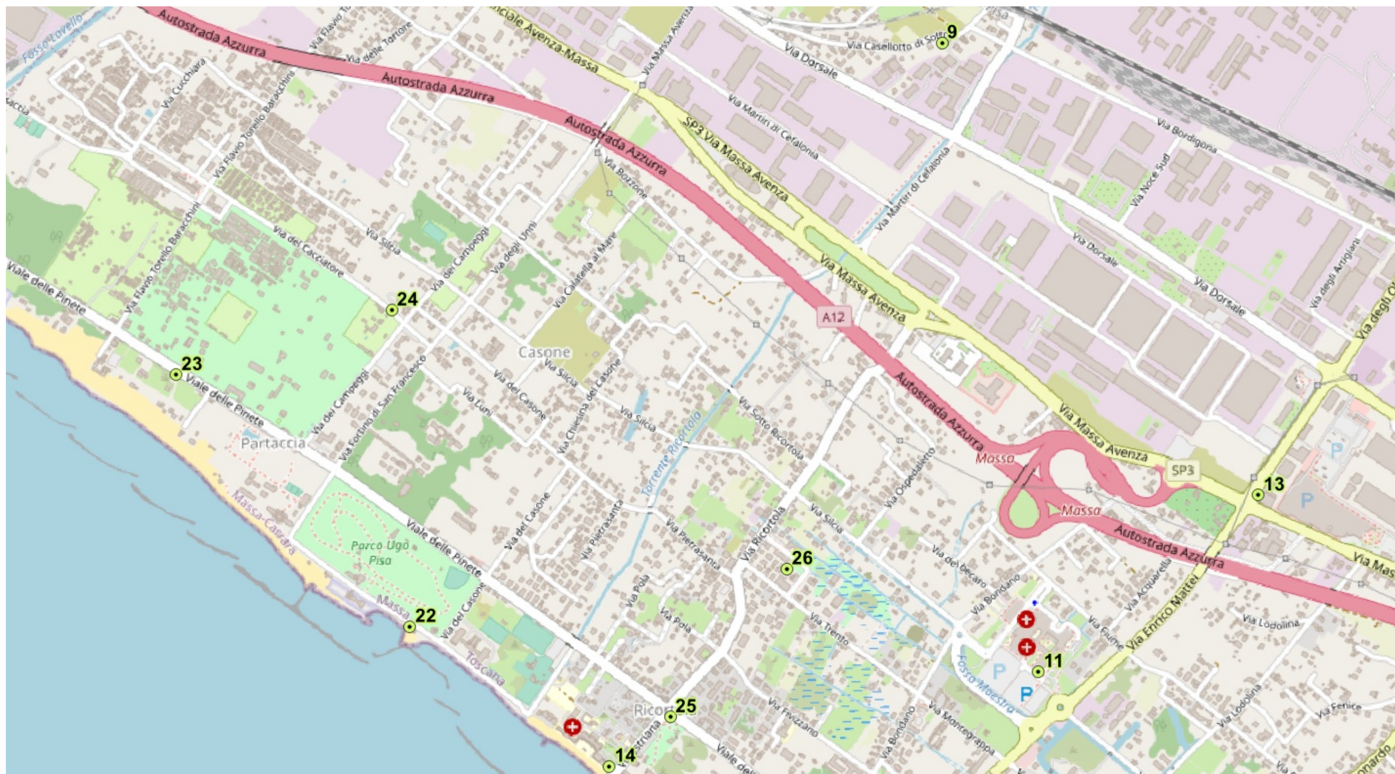
Fig. 4 Individuazione punti di misura – Dettaglio
