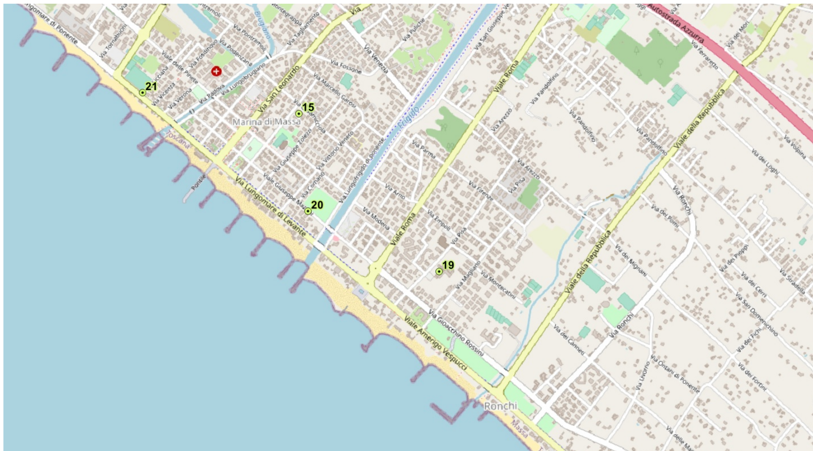
Fig. 5 Individuazione punti di misura – Dettaglio
