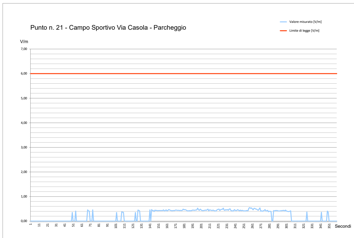
Fig. 70 Grafico Misura di Campo Elettromagnetico a RadioFrequenza – Punto #21
