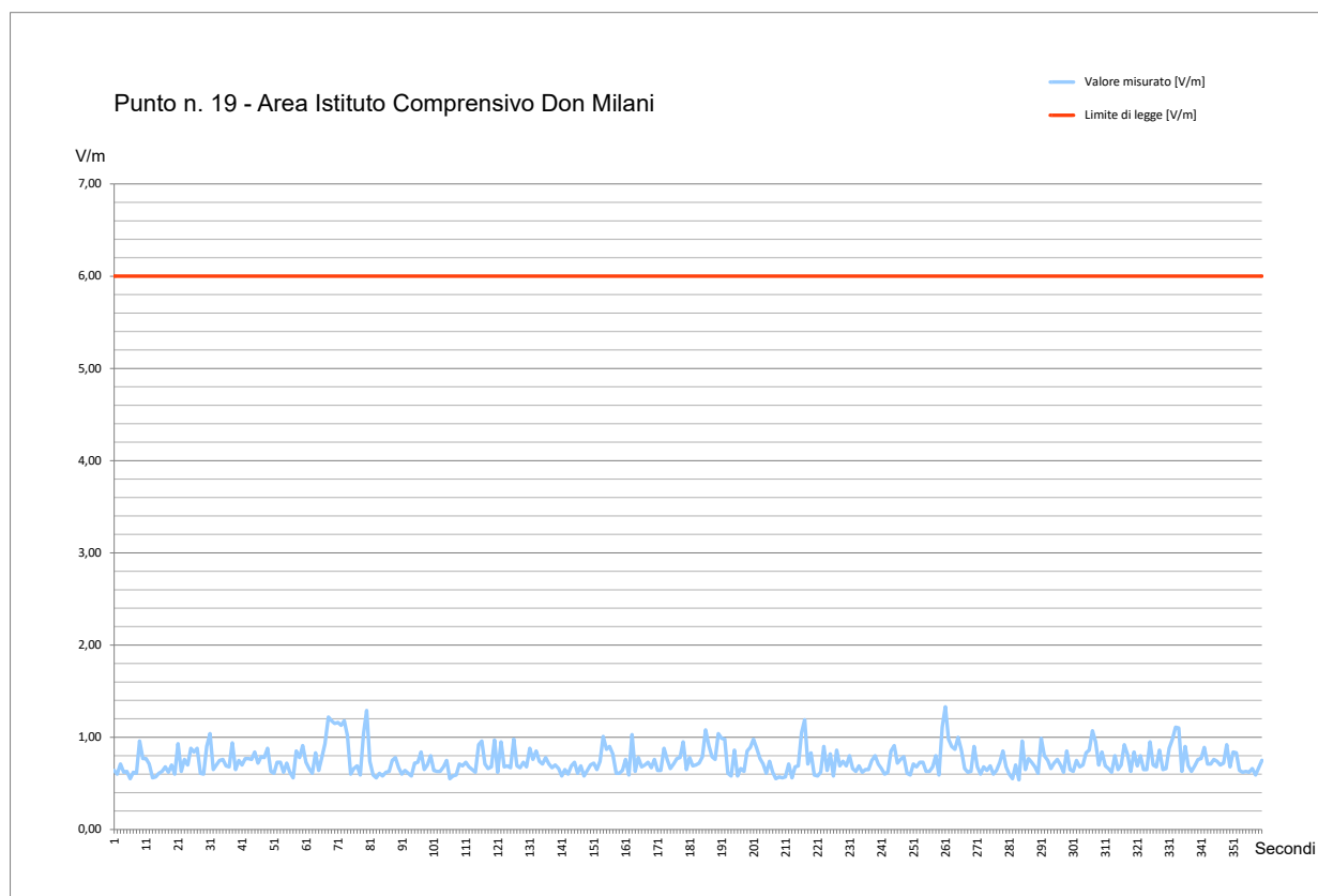
Fig. 64 Grafico Misura di Campo Elettromagnetico a RadioFrequenza – Punto #19
