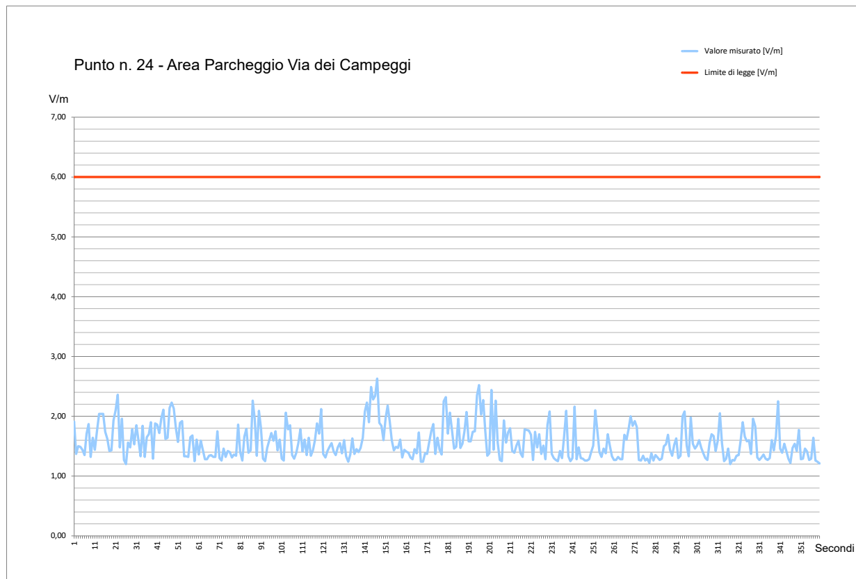
Fig. 79 Grafico Misura di Campo Elettromagnetico a RadioFrequenza – Punto #24
