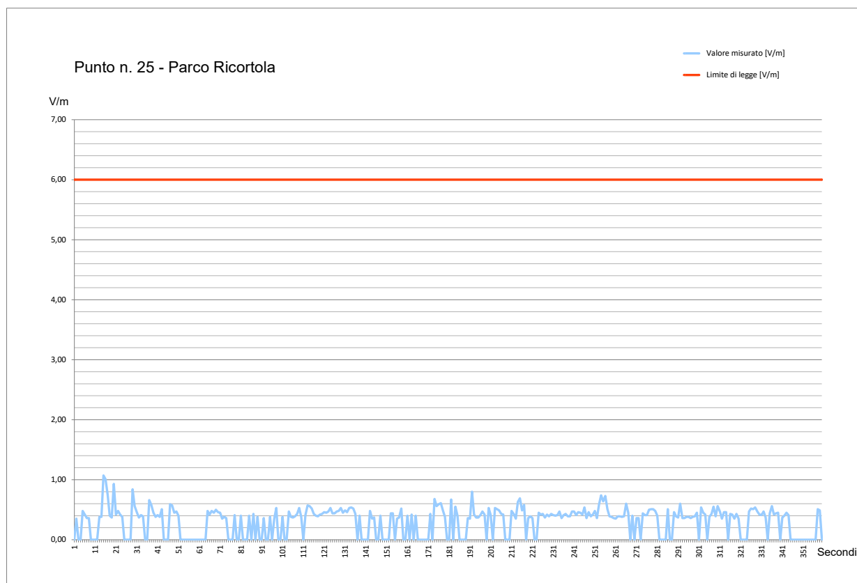
Fig. 82 Grafico Misura di Campo Elettromagnetico a RadioFrequenza – Punto #25
