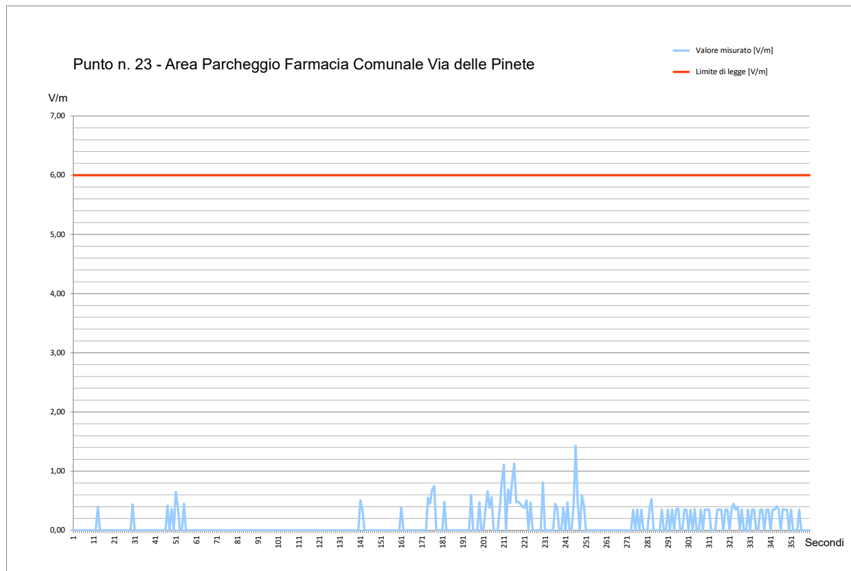
Fig. 76 Grafico Misura di Campo Elettromagnetico a RadioFrequenza – Punto #23
